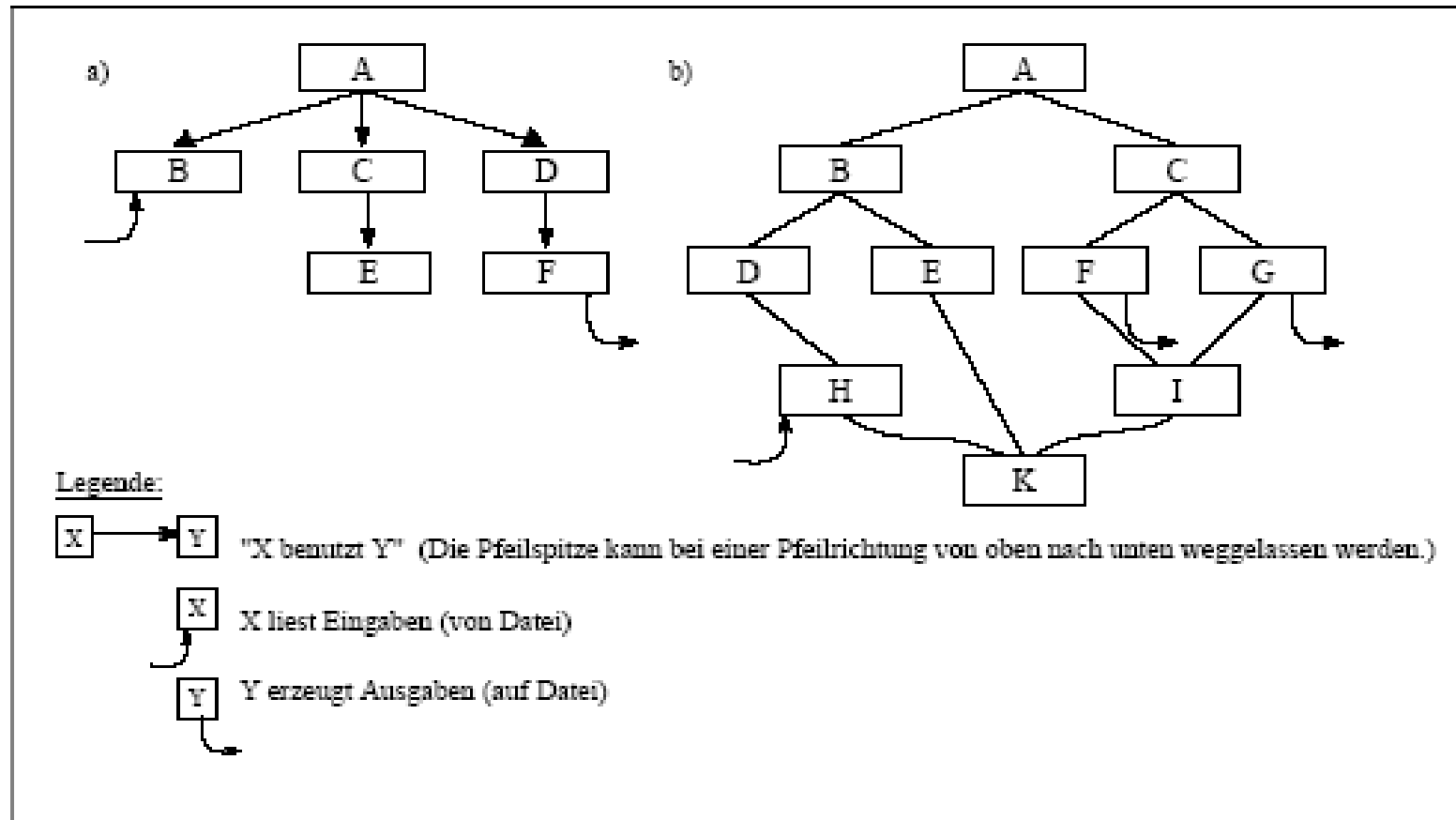
Abb. 13.3: Verschiedene Modulhierarchien
