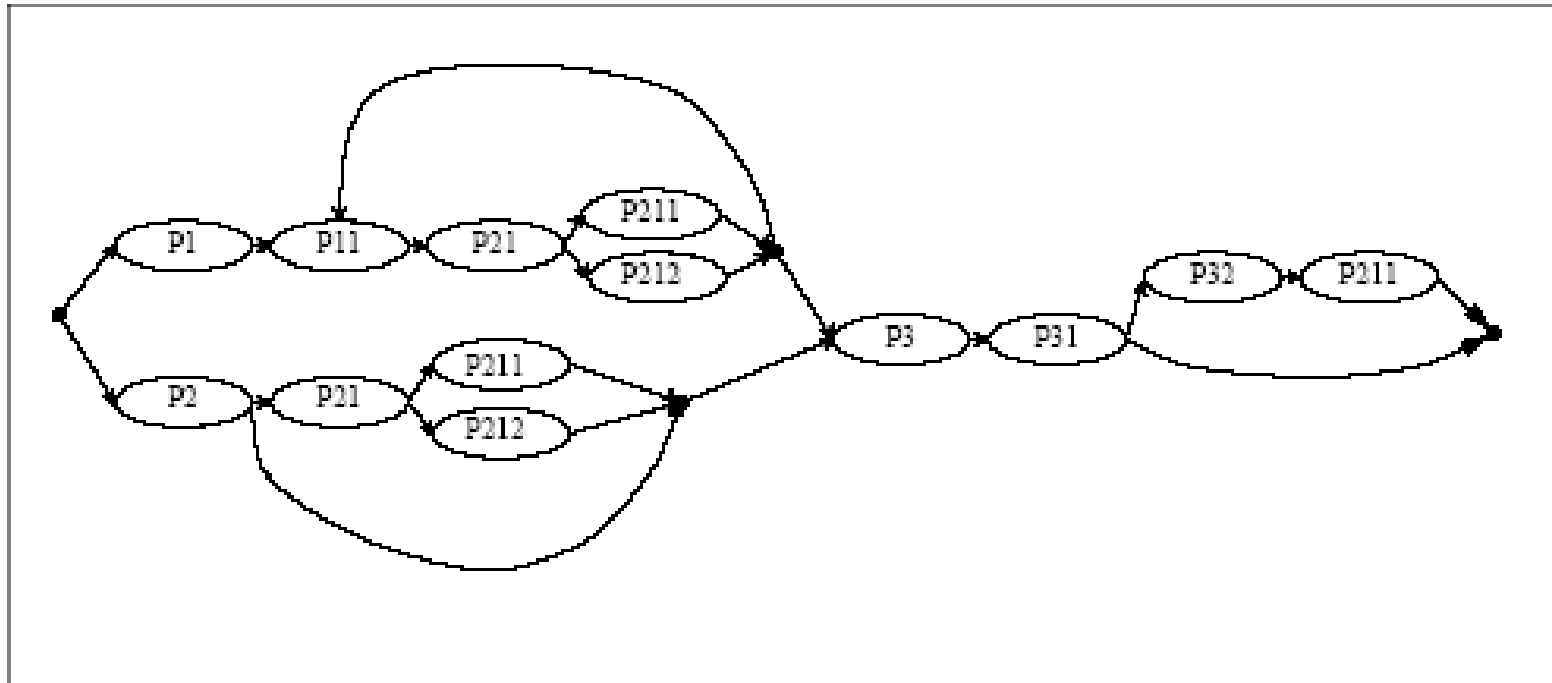
Abb. 13.7: System-Kontrollflußgraph (nach [Spi 90], Abb. 4)
